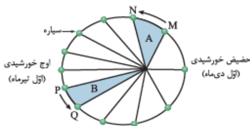
نمایش نظریه خورشیدمرکزی
