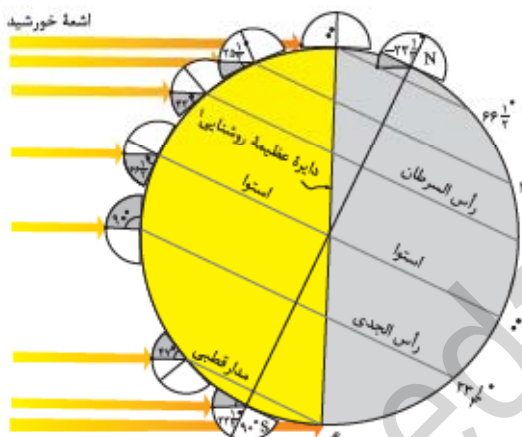
انحراف محور زمین و تاثیر آن در مقدار زاویه تابش خورشید در عرض های جغرافیایی مختلف
