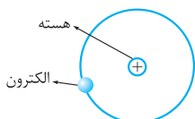
اتم هیدروژن
